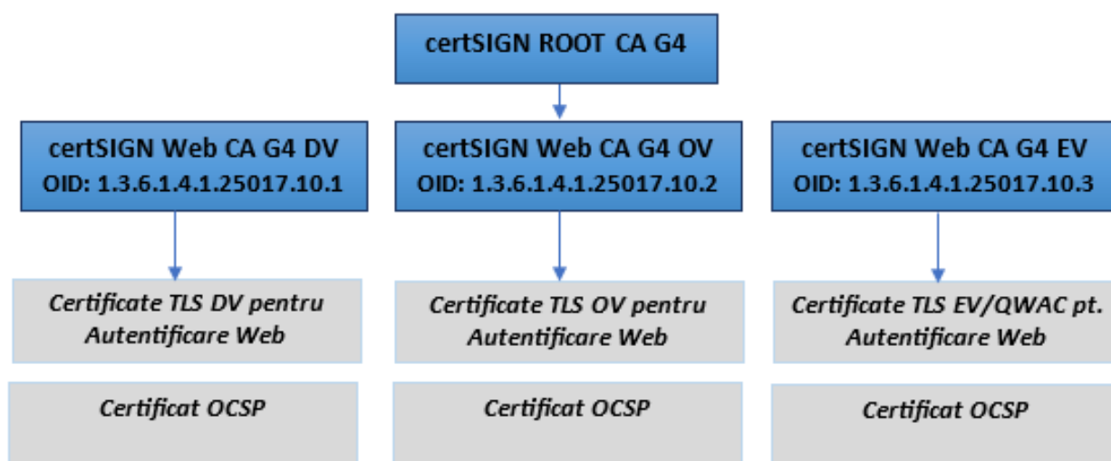
Figure 1: Structura domeniului de certificare certSIGN ROOT CA G4
